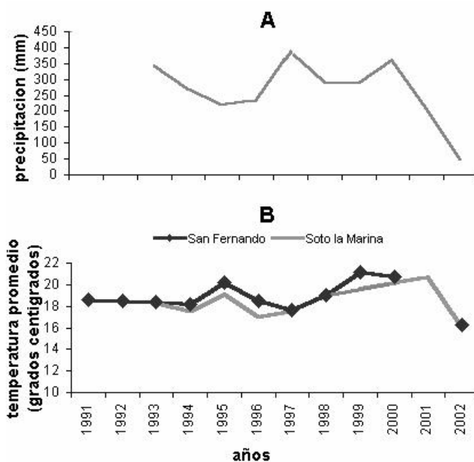
Figura 6. Comportamiento de variables ambientales en la costa de Tamaulipas. a) Precipitación total de noviembre - abril de 1993 - 2002 en la estación de San Fernando, Tamaulipas, b) Temperatura promedio de 1991 - 2002 en las estaciones de San Fernando y Soto La Marina, Tamaulipas. Fuente: Comisión Nacional del Agua.
