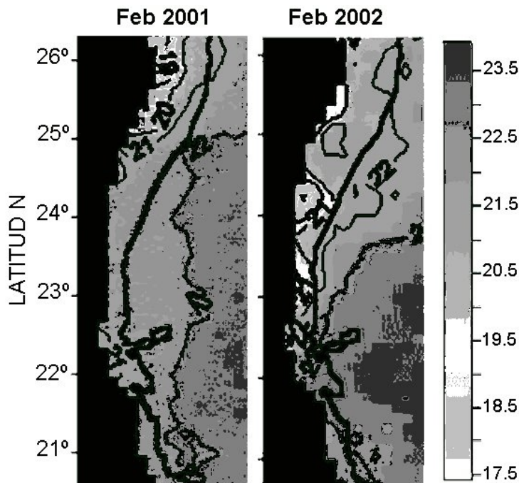
Figura 7. Distribución de la temperatura superficial tomada por satélite en la zona de Tamaulipas en febrero de 2001 y 2002.
